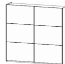
Schwebetürenschränk 2-türig, 1 Einlegeboden und 1 Kleiderstange je Fach B/H/T 218/210/59 cm
